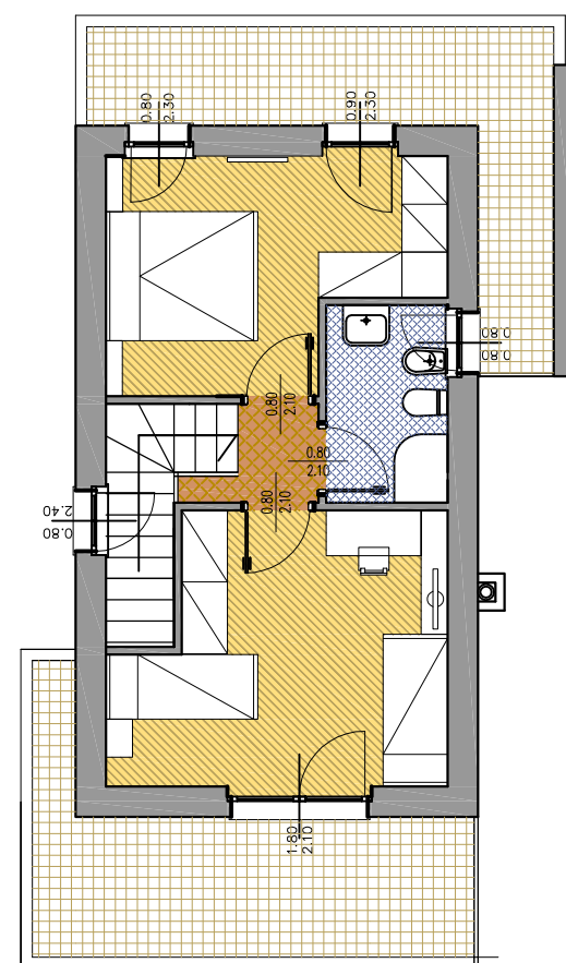
Piano Primo
